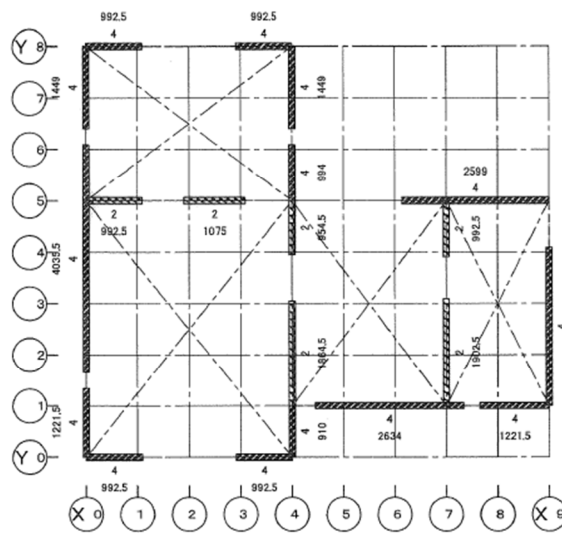
1階耐力壁線図
