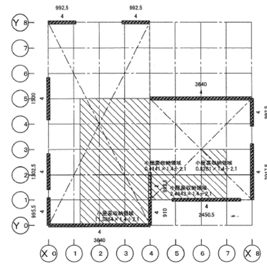
2階耐力壁線図
